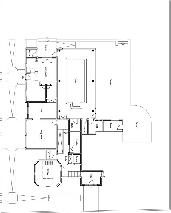
Planta baja
