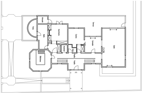
Planta primera
